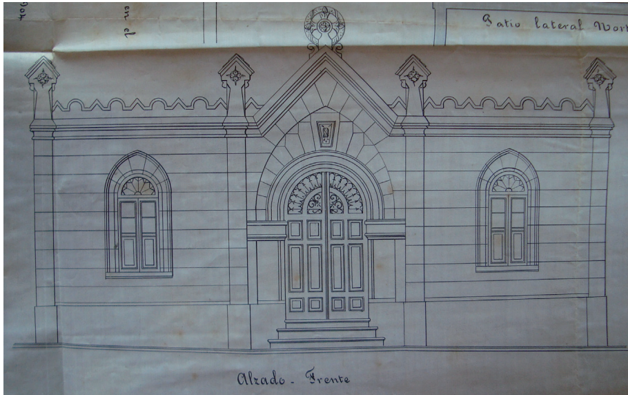
Figura 4. Alzado del proyecto de nueva fachada del cementerio. 1904.
