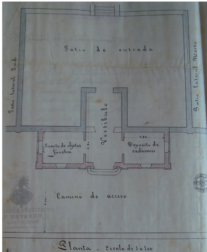
Figura 3. Planta del proyecto de cuerpo exterior de ampliación del cementerio. 1904. Fuente: Archivo Histórico Provincial de Las Palmas.
