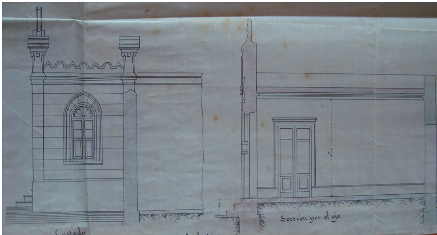
Figura 5. Sección lateral y por el eje del proyecto de cuerpo exterior. 1904. Fuente: Archivo Histórico Provincial de Las Palmas.
