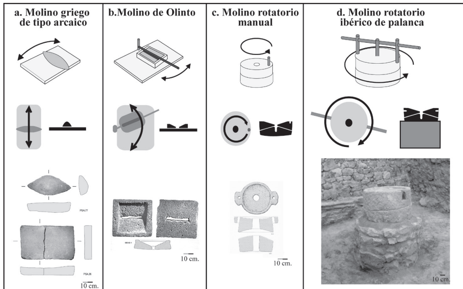
Figura 1. Nuevos tipos de molinos presentes en el Mediterráneo occidental a mediados del primer milenio. (a) Molino griego de tipo arcaico (dibujo inferior, molino de Ullastret, a partir de Portillo, 2006: 29.4); (b) Molino de Olinto (dibujo inferior, molino de Lattara , a partir de Py, 1992: fig. 4); (c) Molino rotatorio manual (dibujo inferior, molino de la Bastida de les Alcusses, a partir de Bonet y Vives-Ferrándiz 2011: fig. 14); (d) Molino rotatorio ibérico de palanca (fotografía inferior, restitución de un molino y su soporte en el Tossal de Sant Miquel, fotografía H.Bonet).
